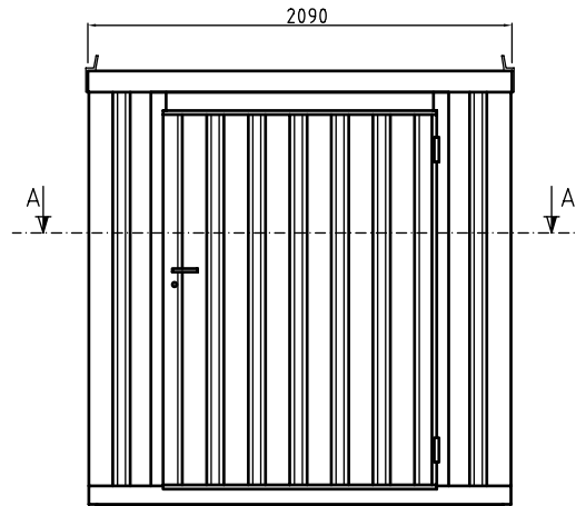
Voor-aanzicht
