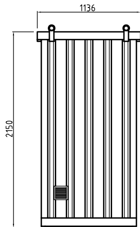
Linker zij-aanzicht
